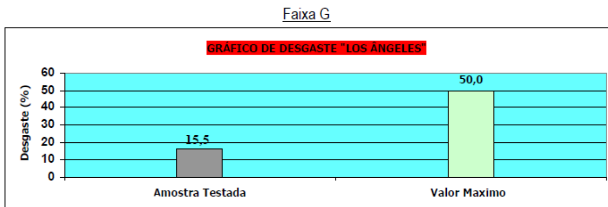
Figura 11 – Ensaio de qualidade da rocha extraída na Pedreira CH Mineração
